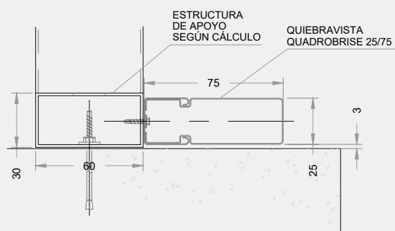
DETALLE INFERIOR
