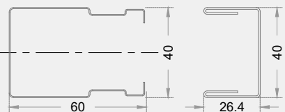
QUADROBRISE 40/60
