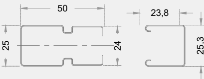
QUADROBRISE 25/50
