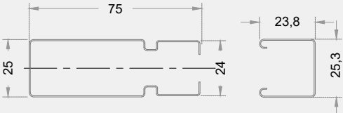
QUADROBRISE 25/75
