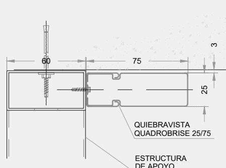
DETALLE SUPERIOR
