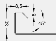
CORTE B-B
